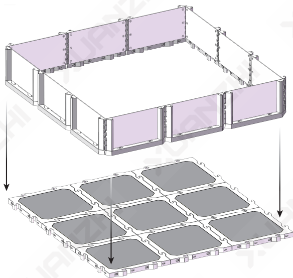
⑥ 将12片拼合好的围栏和底板进行组合
