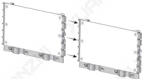
④ 将12块下层围栏拼在一起
