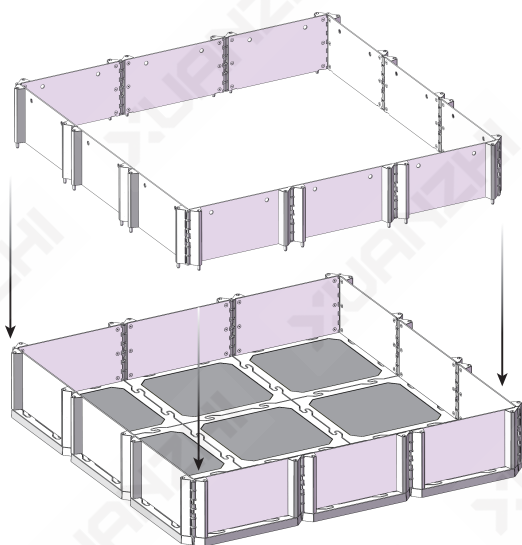
⑩ 将12块拼合好的围栏和第⑦步的组件进行组合
